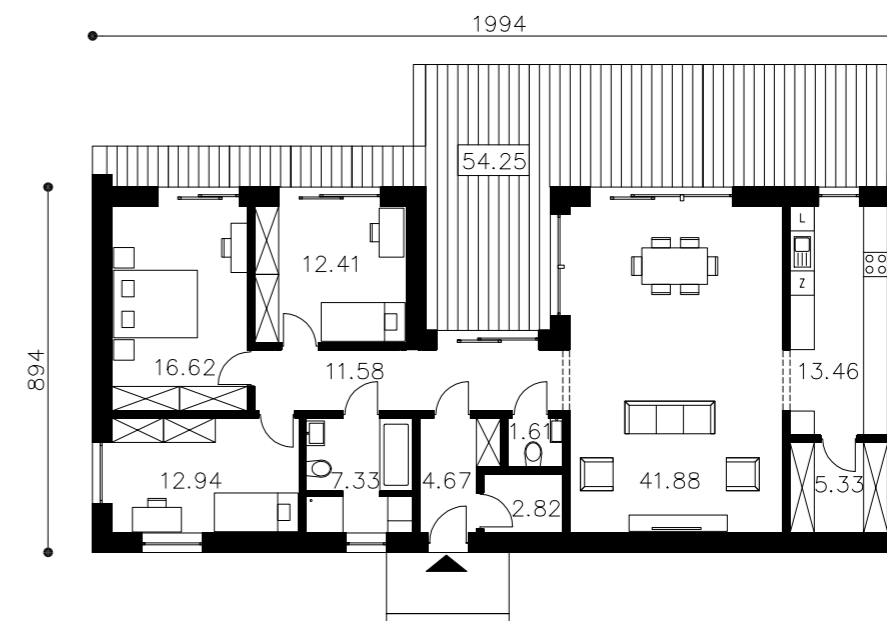
RZUT PARTERU
